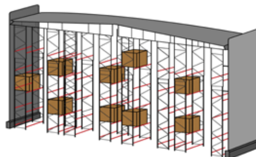
Máxima capacidad de resistencia
