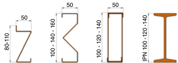
Secciones de vigas para distintas cargas
