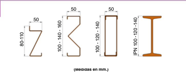
Secciones de vigas para distintas cargas
